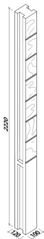
Obr. č. 15 – Nová Trója sloupek průběžný 160, 210, 260, 310
