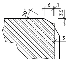
Řez hranou (v 60 mm)
